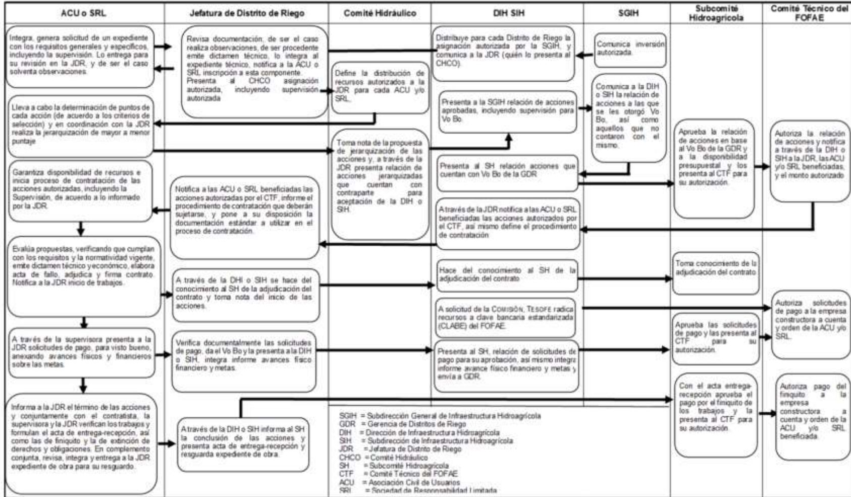
Diagramas de flujo de las componentes del Programa de Apoyo a la Infraestructura Hidroagrícola. Componente para la rehabilitación y tecnificación de distritos de riego modalidad FOFAE
